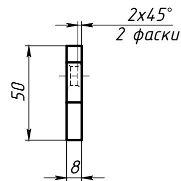
Поз.1 (Проушина)
