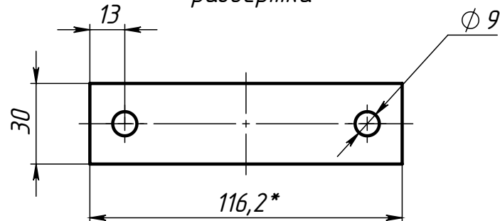
Поз.5 (Полухомут) развертка
