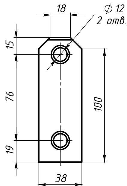
Поз.4 (Серьга)
