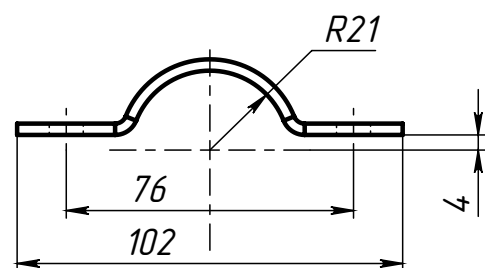
Поз.5 (Полухомут)
