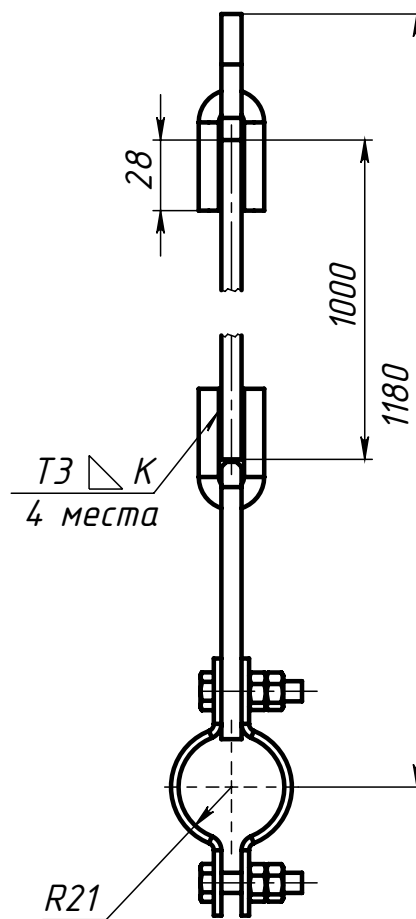
Поз.5 (Полухомут)
