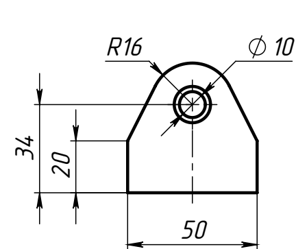
Поз.1 (Проушина)
